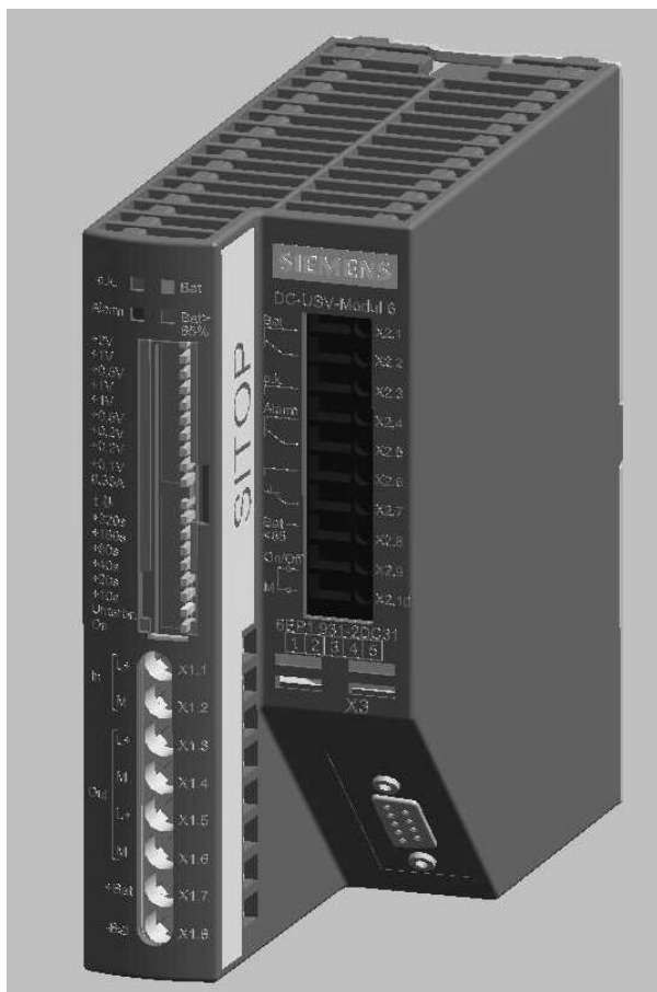
6EP1931-2DC31
